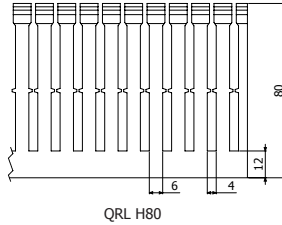
QRL H80
