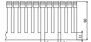
QRL H60
